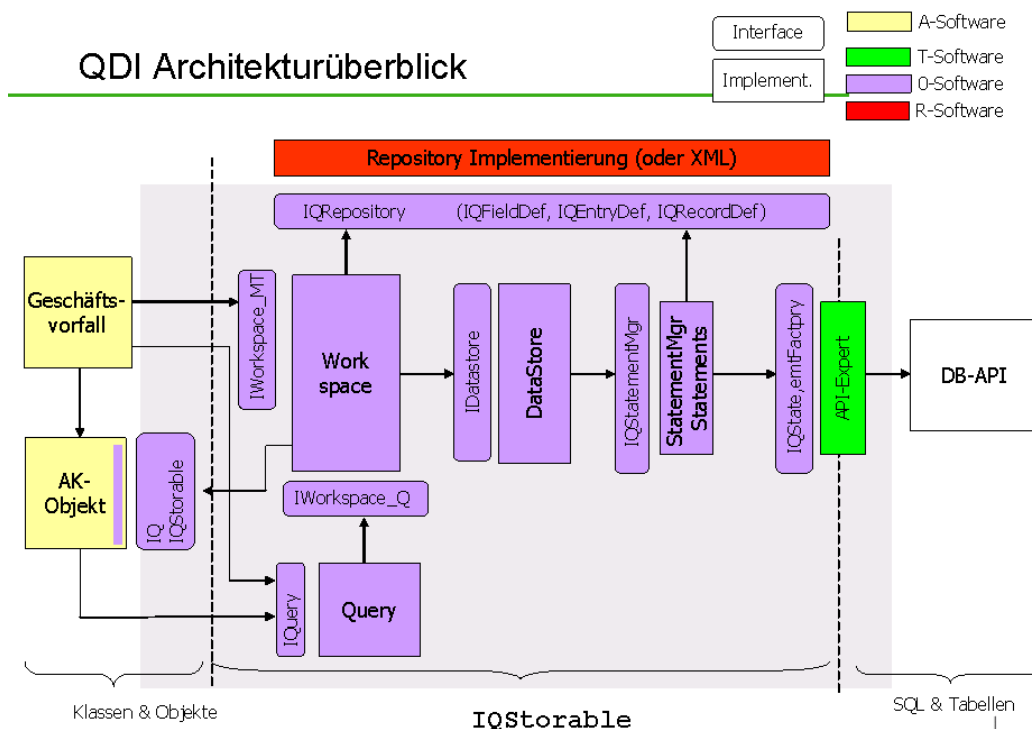
Abbildung 1: Architektur des Quasar-Datenbank-Interfaces, sd&m AG 2001
